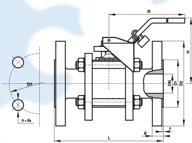
Z zabezpieczeniem przed zaknięciem i otwarciem
