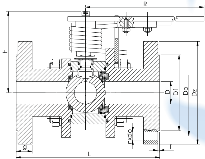
Z zamknięciem/otwarciem za pomocą sprężyny
